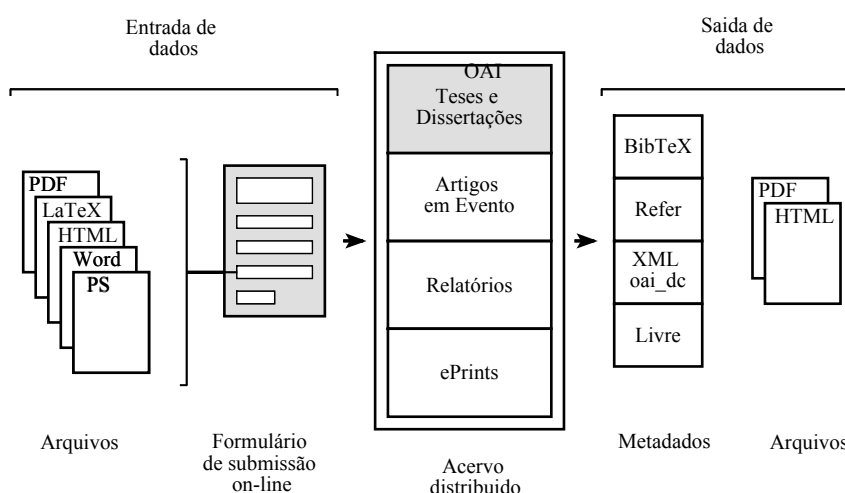
Fig. 4 - Formatos de entrada e saída.
