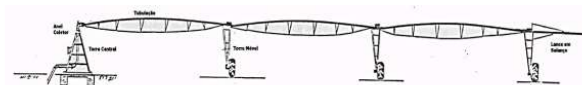
Figura 79: Vista lateral esquemática de um pivô central salientando partes do equipamento.
