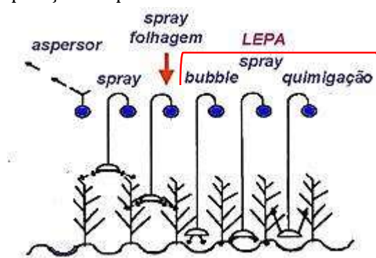
Figura 91: Esquema comparativo dos tipos de emissores utilizados em pivôs e os correspondentes locais de instalação.
