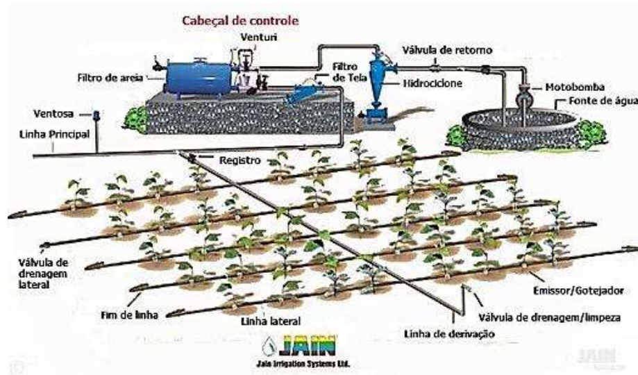
Figura 122: Esquema de um sistema de irrigação localizada em operação no campo (Fonte: JAIN, 2010).
