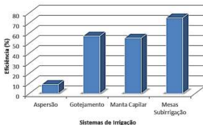
Figura 220: Eficiência de aplicação em sistemas de irrigação utilizados em cultivos de vasos (Fonte: NEAL et al., 1995).
